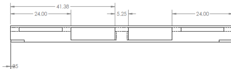
Рисунок 2 Габариты длинной стороны поддона
