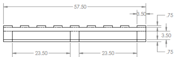
Рисунок 3 Габариты короткой стороны поддона
