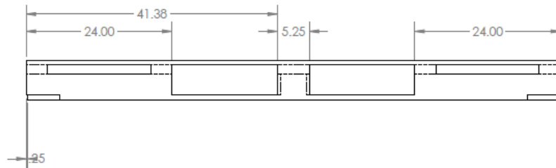
Rys. 2 Wymiary dłuższej strony palety
