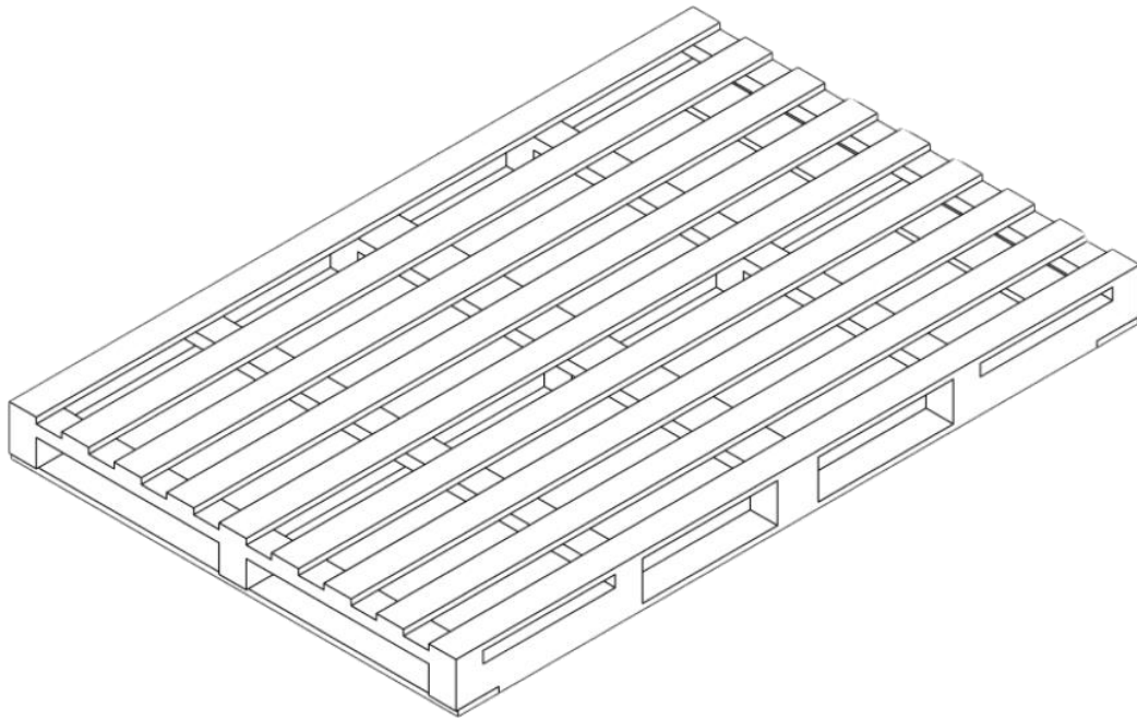
Rys. 1 Schemat nowej palety na płyty o wymiarach 50x80 i 50x65
