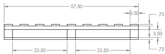
Rys. 3 Wymiary krótszej strony palety
