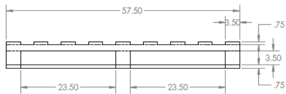
Abbildung 3 Abmessungen der kurzen Seite der Palette
